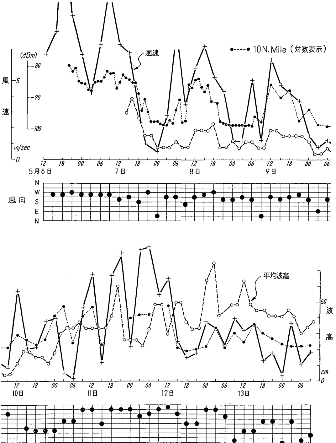
第3図 紋別沖北東10渚点からの反射電力と波高・風との関係 (1969年5月6日~13日)
