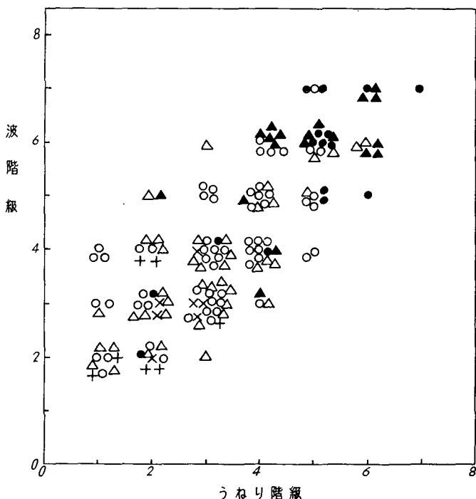
第4図 波浪階級・うねり階級としづき量の関係
