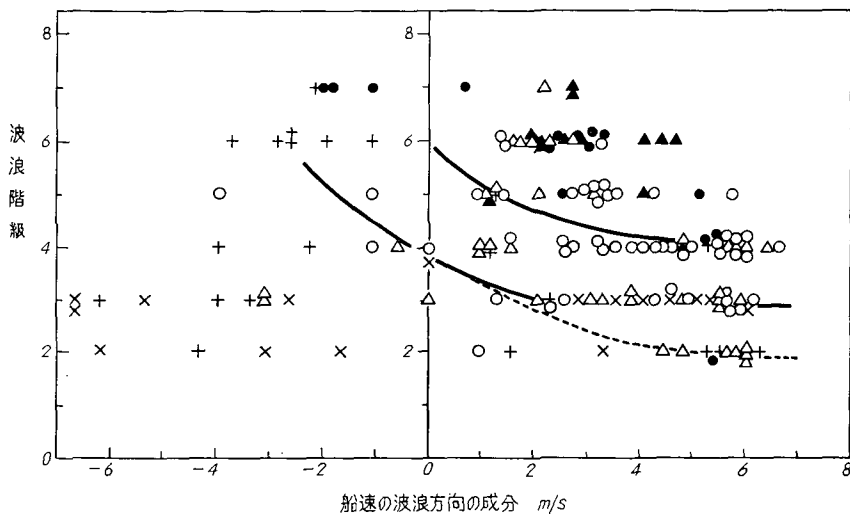
第3図 船の速さの波浪方向の成分・波浪階級としづき量の関係
