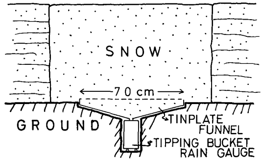
第1図 融雪滲透水の測定装置
