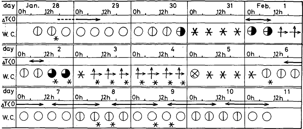
第4図 観測期間中の天気状況と盆地冷却発生時間
