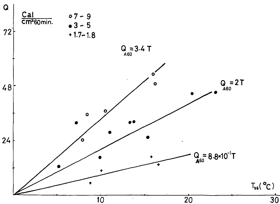
第8図 頭熱伝達量 Q_A と風洞中心の気温 T_{25} との関係
