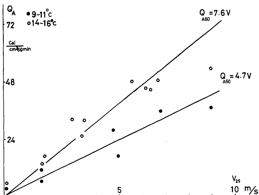
第7図 頭熱伝達量 Q_A と風洞の中心風速 V_{25} との関係
