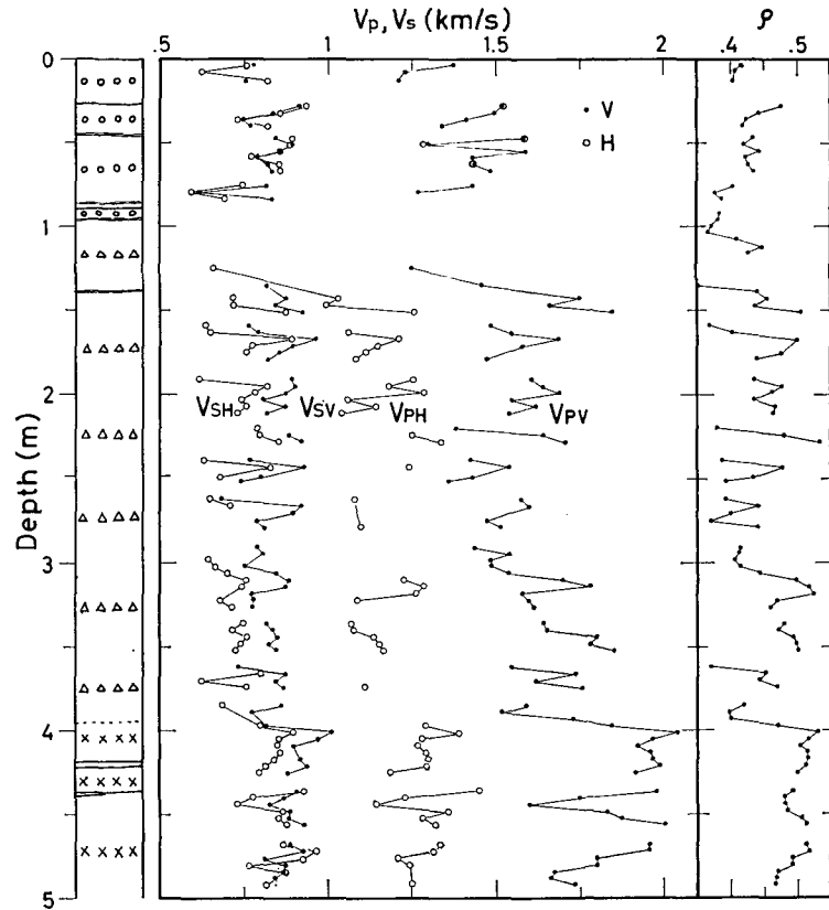
第2図 表面から深さ5mまでの雪質と V_{SH}, V_{SV}, V_{PH}, V_{PV} , 密度 ( \rho ) の分布。雪質分布図で○はしまり雪, △はしもぎらめ雪, ×は圧密雪である。 V_P, V_S の分布図で○は水平方向。●は鉛直方向の V_P, V_S である。
