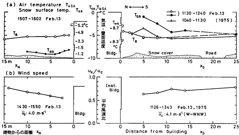
第9図 (a) 融雪が無い時期(2月13日)における低温科学研究所の建物の南北の気温 T_{a,0.4} (雪面上40cm) および雪面温度 T_{ss} の分布の観測例。 図中、建物の内側に記載した温度は外壁表面の放射温度 (b) 建物の南北における平均風速 \bar{u}_x の分布。建物の影響が無い場所の平均風速 \bar{u}_c との比、高さは雪面上50cm
