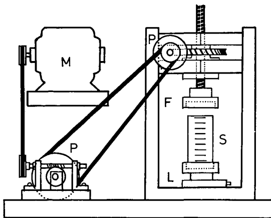
第1図 実験装置の略図
