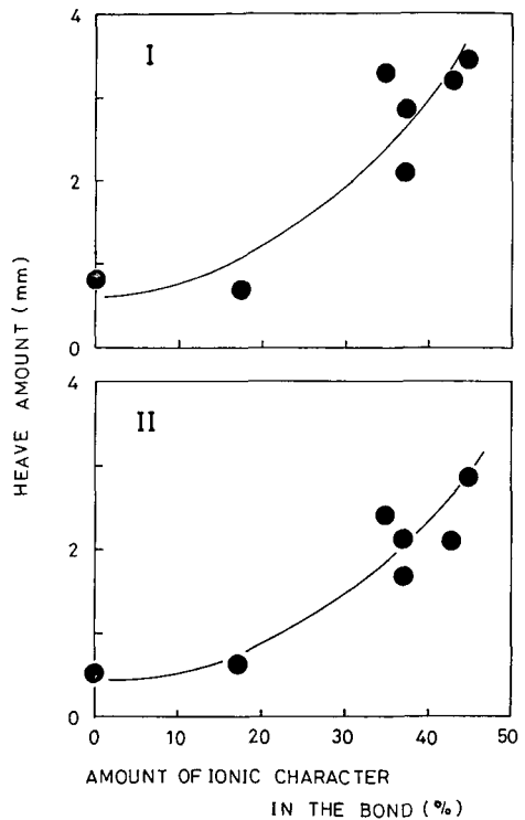
第2図 凍上量と化学結合中イオン性結合の占める割合(%)との関係。Ⅰは冷媒の温度が -15^{\circ}\text{C} , Ⅱは冷媒の温度が -30^{\circ}\text{C}
