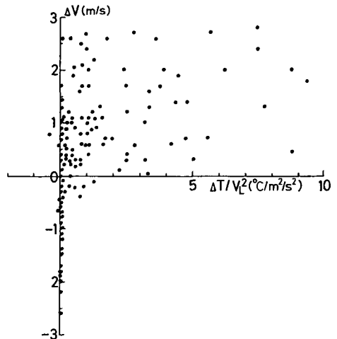
第 6 図 山頂と盆地における風速差と安定比の関係
