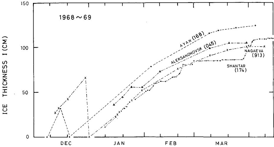
第2図 1968~'69年の氷厚増加の例
