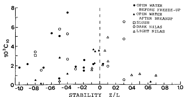
第5図 抵抗係数 ( 10^3 C_{10} ) と安定度 ( z/L ) の関係
