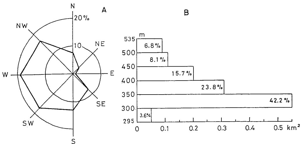
第2図 全流域面積に占める斜面方位別面積(A)と高度別面積(B)の割合
