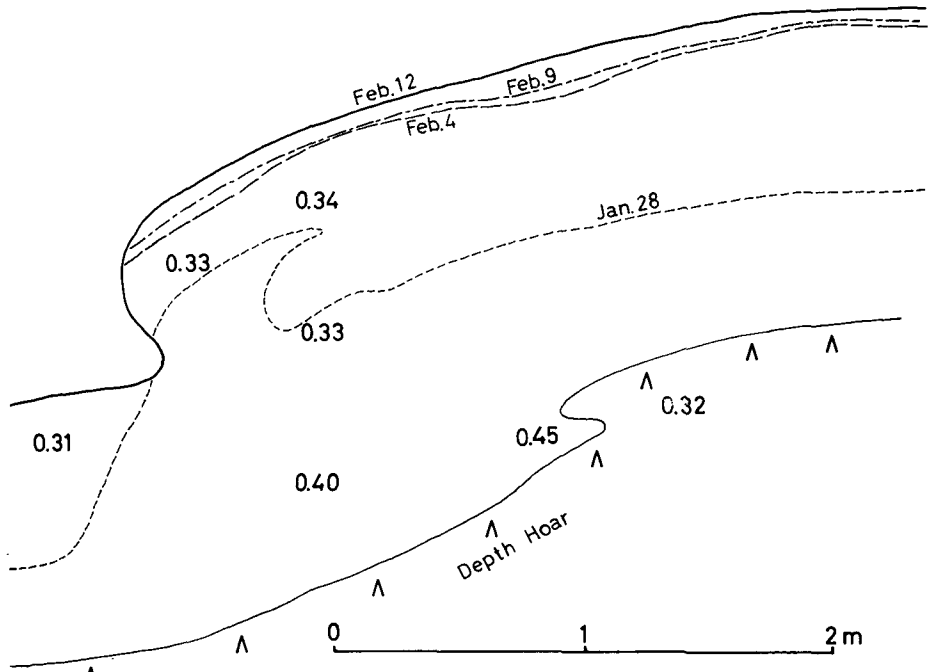
第3図 観測点Jの雪庇の、J-K方向の断面図(1972年2月12日) 各層に記された日付は色水散布した月日で、その時の雪庇表面を示している。 各層間の数字は積雪の密度 ( \text{g}/\text{cm}^3 )
