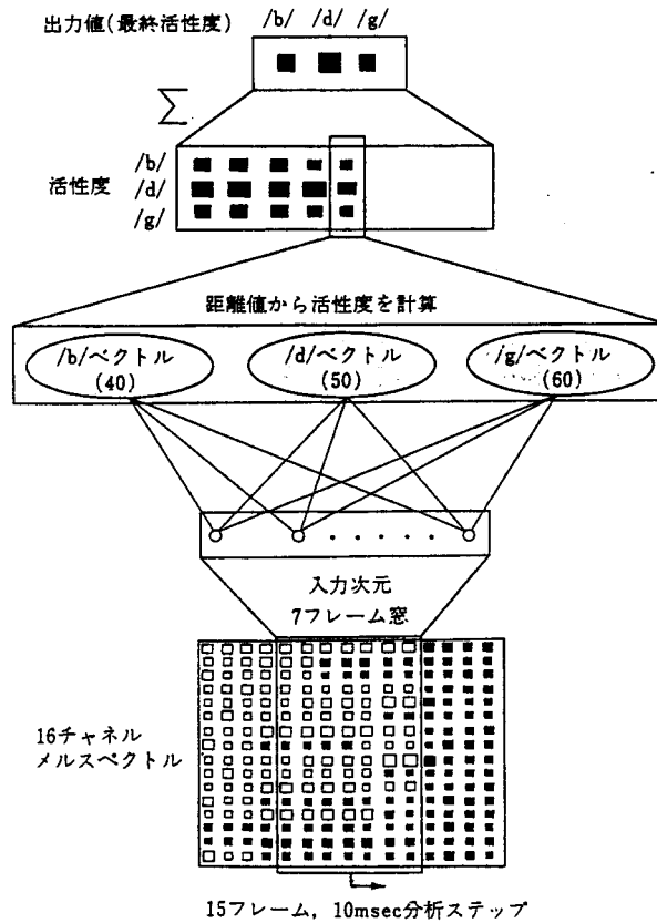
図 22: Shift-Tolerant-LVQ の構造 (鹿野他 [2])
