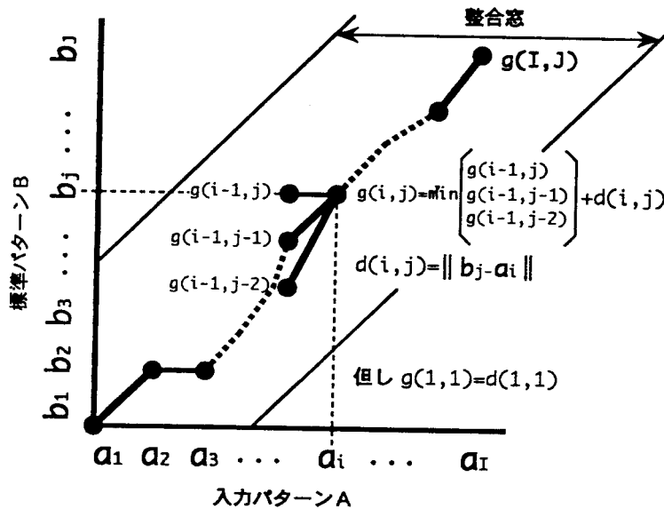
図 16: 動的計画法を用いた時間軸の適応正規化の一例 (中川他 [2] を修正)
