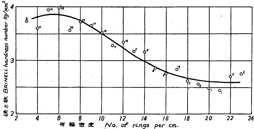
■ 4 芦別産ミズナラの気乾材 (含水率 15%) における年輪密度と硬さとの関係
