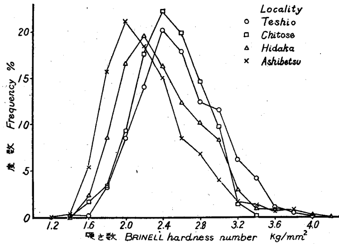
圖 7 硬さ数の出現度数
