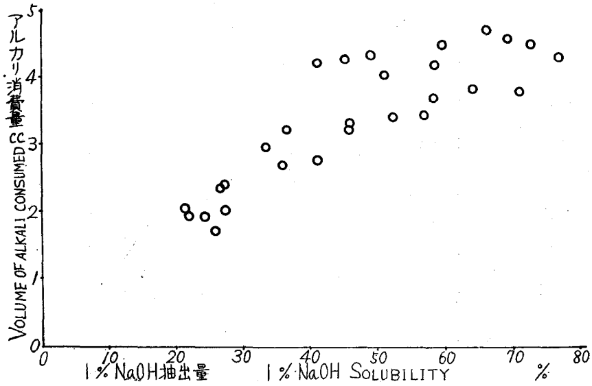
第10図 針葉樹腐朽材のアルカリ消費量と1% NaOH 抽出物との関係
