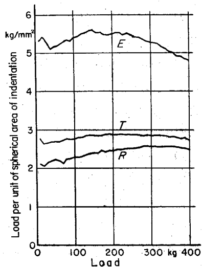
第7図 前図と同じ試験における荷重と BRINELL 硬さ数との関係
