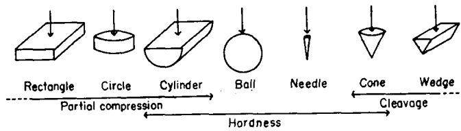
第1図 静的押しつけ硬さ試験の種類
