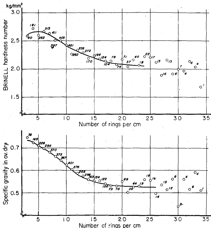
第23図 ミズナラ材における年輪密度と木口面硬さ(生材)および全乾比重との関係
