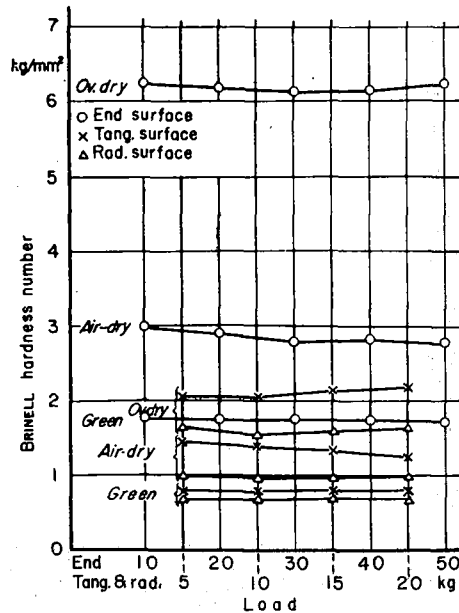
第5図 荷重とBRINELL硬さ数との関係 (ミズナラ材)
