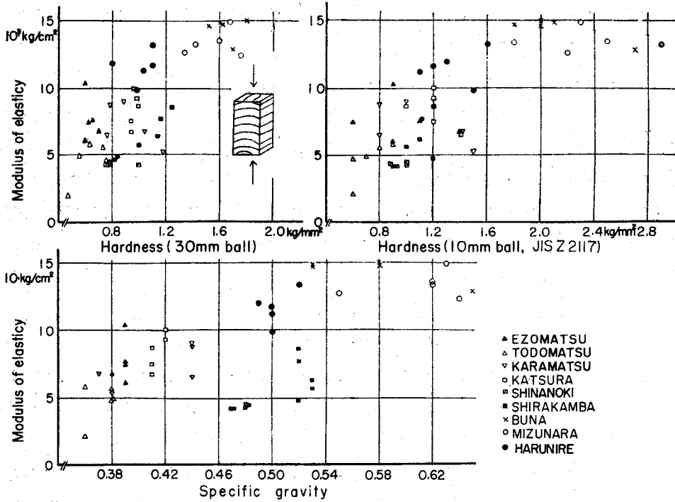
第31図 板目面硬さおよび比重とまさ目方向の横圧縮ヤング係数との関係
