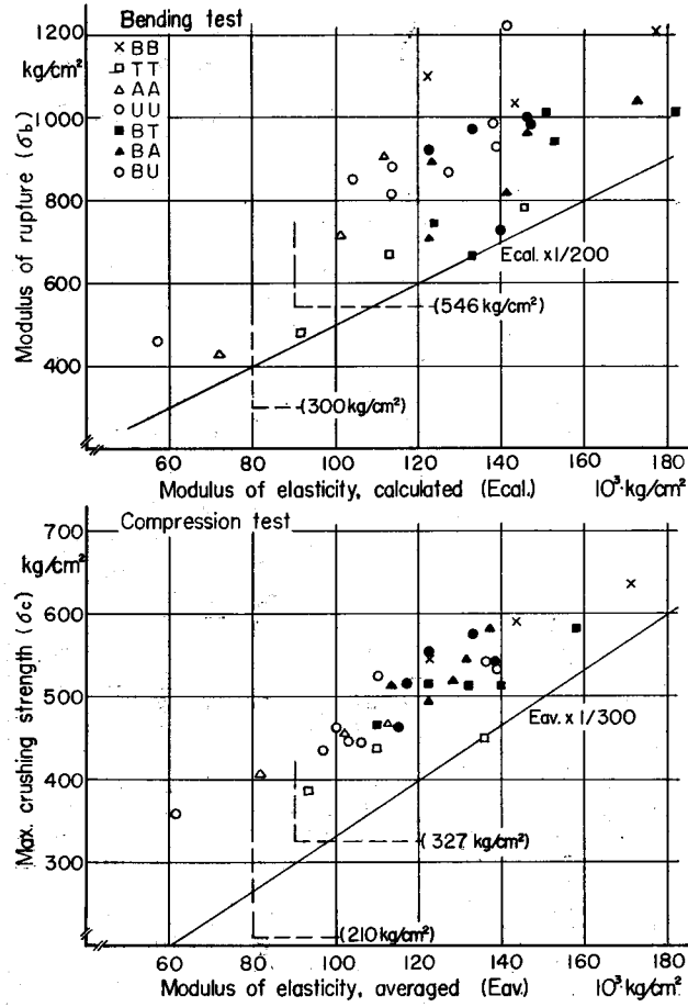
図10. ヤング係数(計算値)と強度との関係
