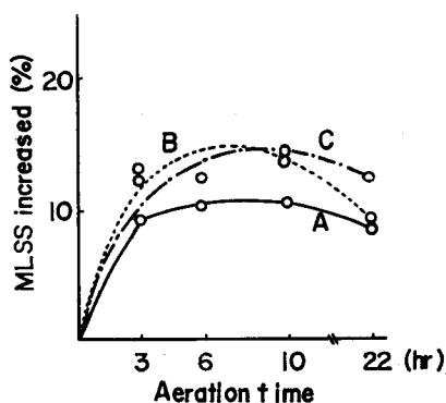
図-7 栄養塩類添加量の相違による曝気時間と MLSS 増加率の関係
