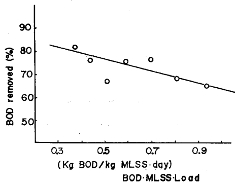
図—3 BOD・MLSS 負荷と BOD 除去率との関係
