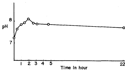
図-10 活性汚泥処理中における pH の挙動
