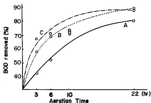
図—5 栄養塩類添加量の相違による曝気時間と BOD 除去率との関係
