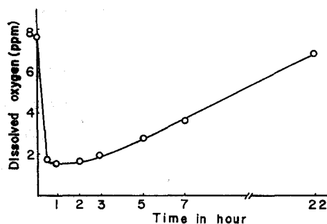
図-11 活性汚泥処理中における溶存酸素の挙動
