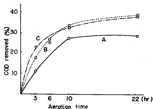
図—6 栄養塩類添加量の相違による曝気時間と COD 除去率との関係
