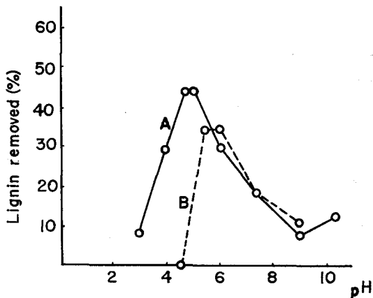
図-14 塩化アルミニウムによる凝集時の pH がリグニン除去に及ぼす影響
