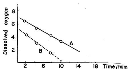
図-2 酸素消費速度 (順養5日目)
