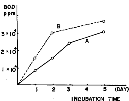
図-1 順養期における BOD 曲線
