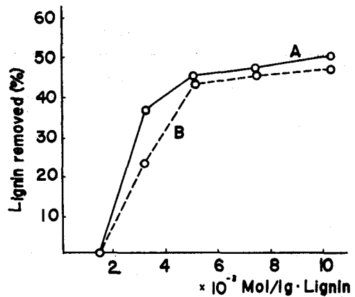
図-13 硫酸アルミニウム添加量とリグニン除去率との関係
