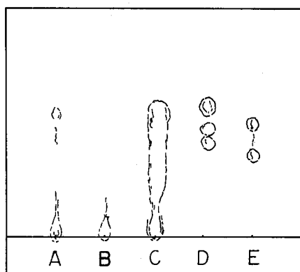
図-8 PPC による廃液中の糖類の挙動
