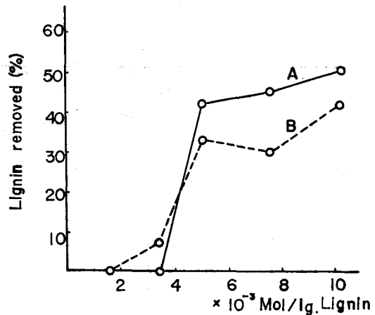
図-15 塩化アルミニウム添加量とリグニン除去率との関係
