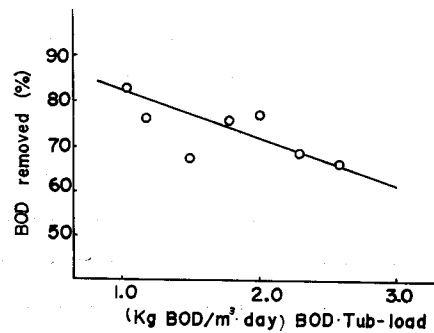
図—4 BOD・槽負荷と BOD 除去率の関係
