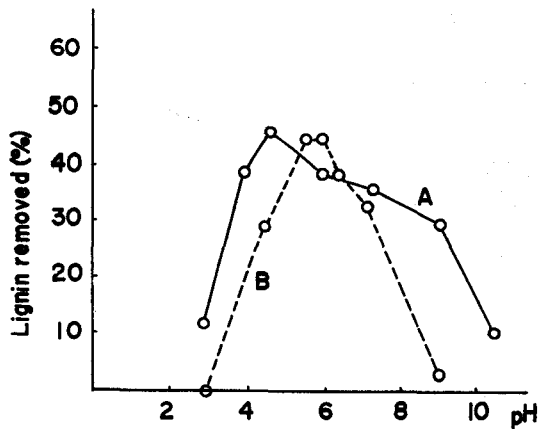
図-12 硫酸アルミニウムによる凝集時の pH がリグニン除去に及ぼす影響
