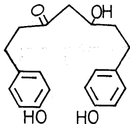
X Platyphyllonol ( Betula platyphylla )
