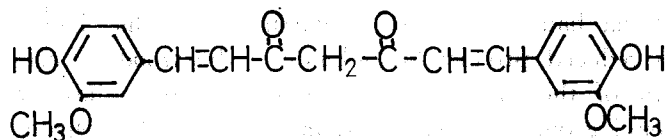
XII Curcumin ( Curcuma : Zingiberaceae)
