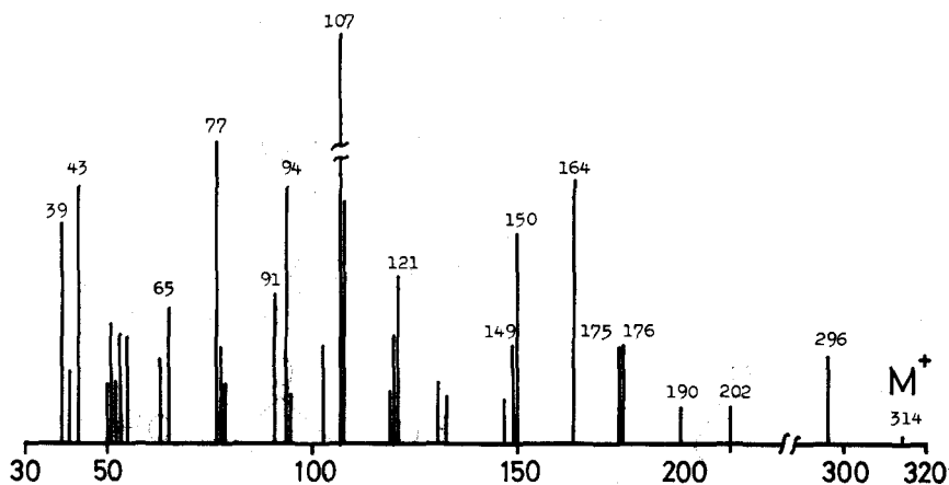
Fig. 20. Mass spectrum of E-4 (1,7-di-( p -hydroxyphenyl)-heptane-3-one-5-ol).
