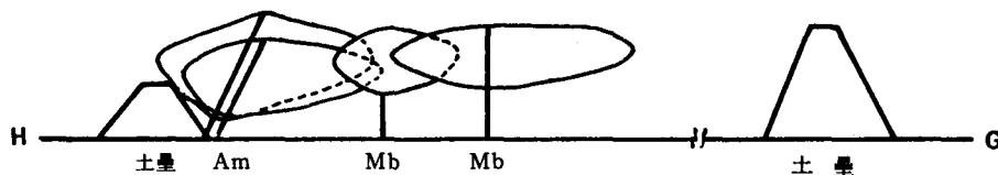
図-37 鷗島調査地2 G~Hの側面図
