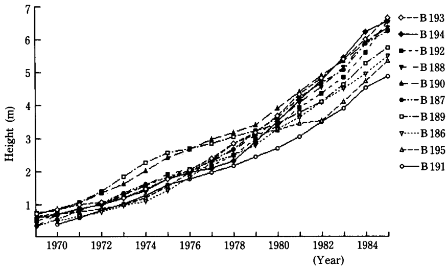
図-9 ストローブマツの樹高成長曲線 Fig. 9. Height growth curve of Pinus strobus .
