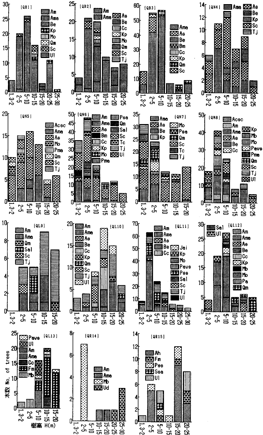
図-7 15調査方形区の樹高階別本数分布図
