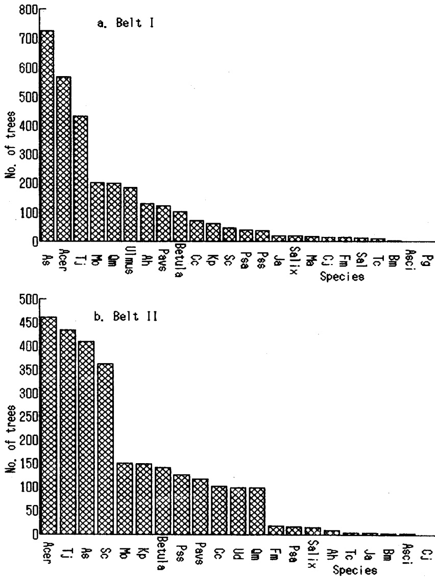
図-17 銅蘭川流域周辺域の帯状区皆伐データによる個体数-種順位曲線
