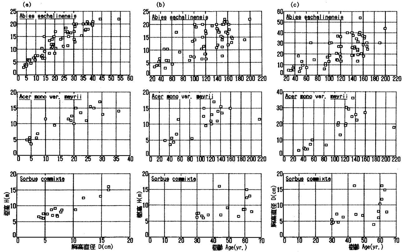
図-16 3調査方形区のトドマツ、アカイタヤ、ナナカマドの胸高直径—樹高、樹齢—樹高、樹齢—胸高直径関係図
