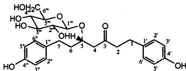
(4) platyphylloside
