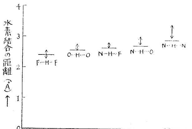
第4圖 水素結合の距離
