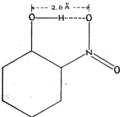
第5圖 オルト・ニトロフェノール
