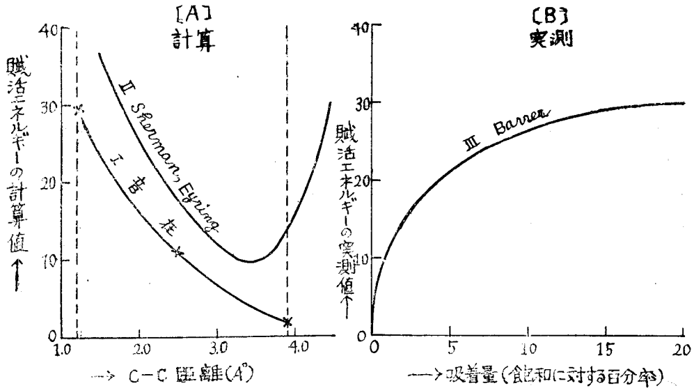
第6圖 木炭に對する水素の解離吸着の賦活エネルギー
