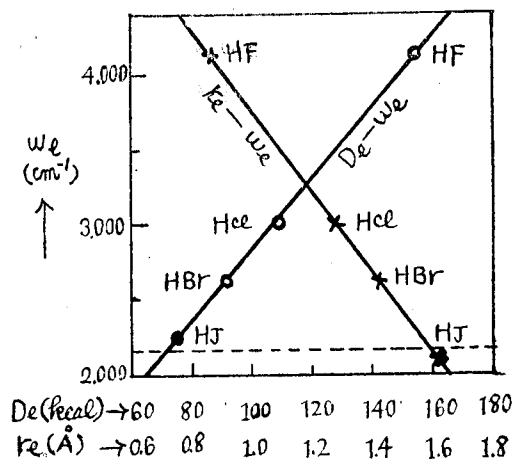
第2圖 HX の \omega_e と D_e , r_e との関係
