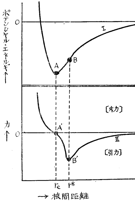
第1圖 二原子分子のポテンシヤル・エネルギー及び力
