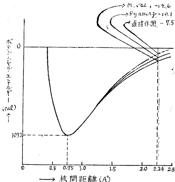
第3圖 H 2 の基底状態のポテンシャル・エネルギー曲線
