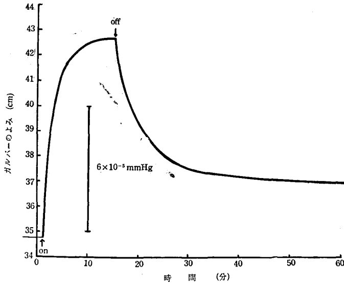
第4図 酸素の光脱離 温度: 18.2°C 平衡圧: 4 \times 10^{-1} mmHg
