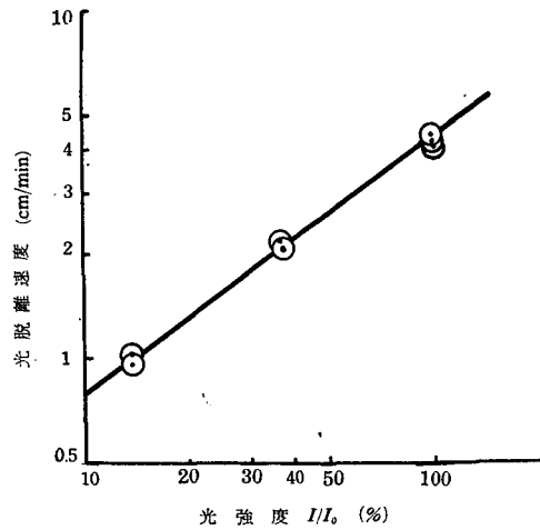
第6図 光脱離初期速度と光強度との関係 条件は第5図と同じ
