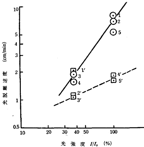
第5図 光脱離初期速度と光強度との関係 温度: 19.3°C 平衡圧: 4.5 \times 10^{-1} mmHg 1 \text{ cm/min} = 1.2 \times 10^{-5} \text{ mmHg/min}
