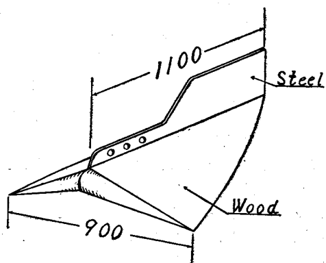
Fig. 3 Depressor
