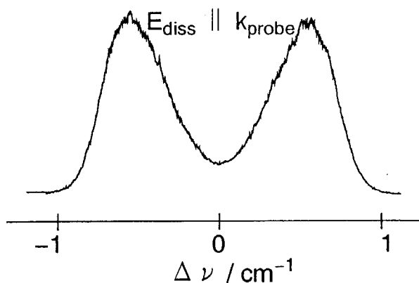
図1 酸素分子 O_2 の157 nm 光分解で生成する酸素原子 O(^1D) の真空紫外レーザー誘起ケイ光ドップラー波形スペクトル。
