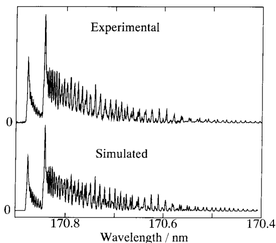
図1 ClOラジカル C^2\Sigma^- - X^2\Pi(v' = 0 - v'' = 0) のレーザー励起スペクトル。上段は実験結果、下段は300 Kの回転温度を仮定したシミュレーション。
