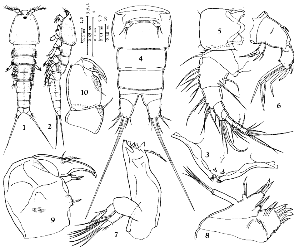
Fig. 3. Paratigriopus hoshidei n. gen. et sp. 1. ♀, dorsal; 2. ♀, lateral; 3. ♀, labrum; 4. ♀, abdomen; 5. ♀, antennule and rostrum; 6. ♀, antenna; 7. ♀, mandible; 8. ♀, maxillula; 9. ♀, maxilla; 10. ♀, maxillipede.
