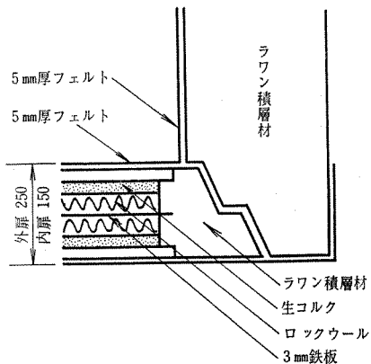
B-4 図 シールド室外扉と内扉の構造
