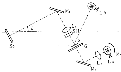
A-6 図 刺戟投射光学系
