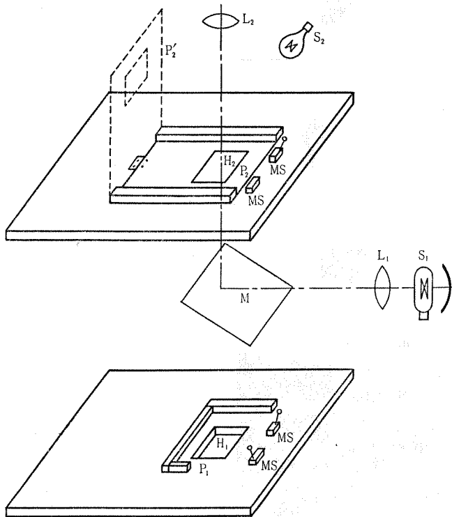
第3-7図 刺戟投射装置
