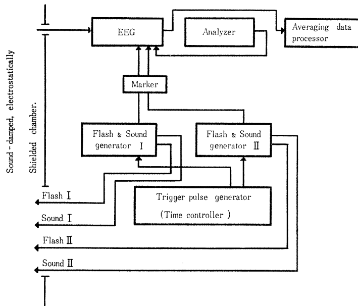
B-5 図 実験室設備ブロックダイアグラム (II) Audio 設備の一部はブロックダイアグラム (I) を参照。
