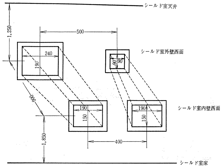
B-6 図 シールド室埋め込み刺戟投射孔
