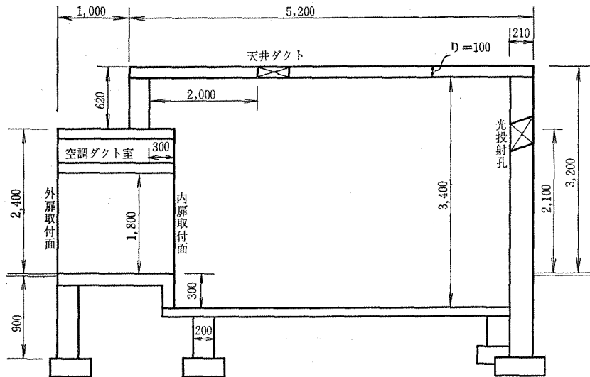
A-1 図 旧シールド室側面図
