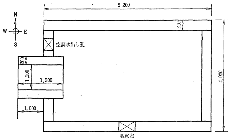
A-2 図 旧シールド室平面図
