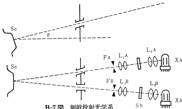
B-7 図 刺戟投射光学系
