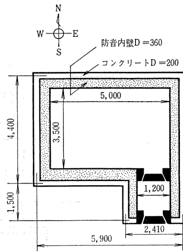
B-1 図 シールド室平面図
