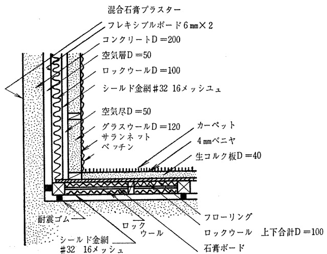
B-3 図 シールド室防音内装の構造
