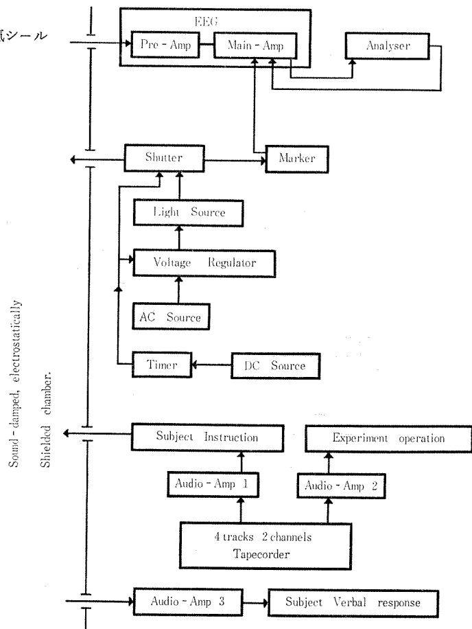
A-5 図 実験室設備ブロックダイアグラムの一例 (I)
