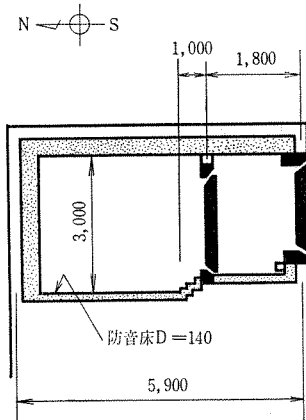
B-2 図 シールド室側面図
