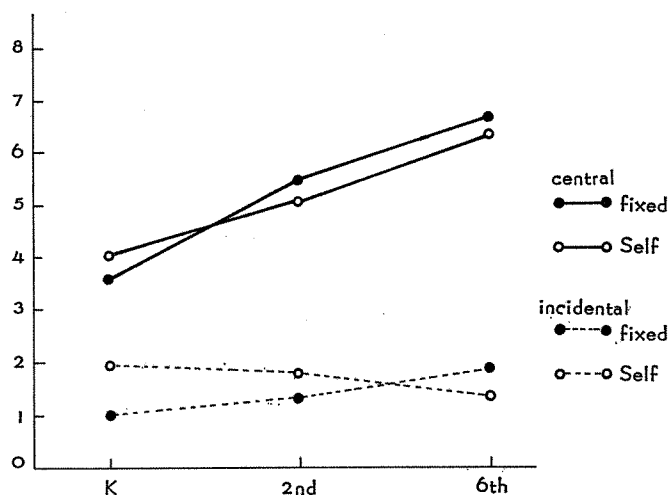
Fig. 2. 平均再生数
