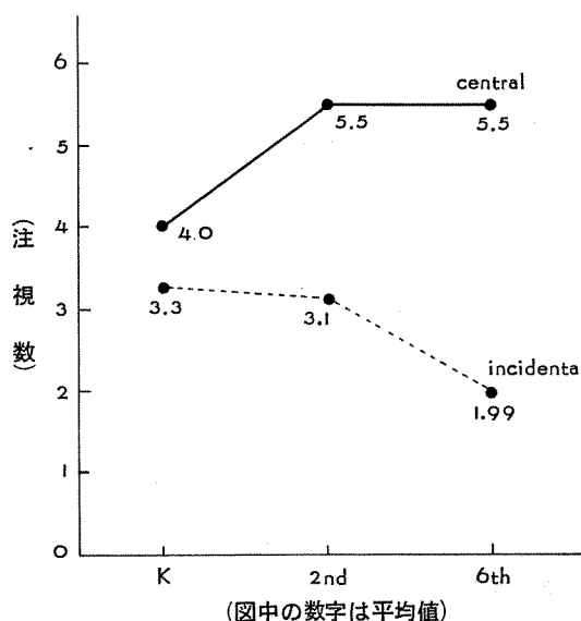
Fig. 3. 平均注視点
