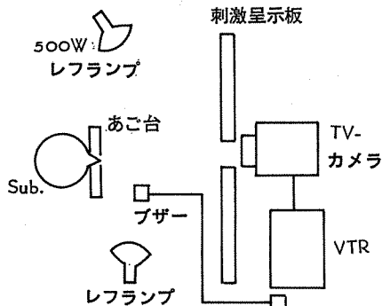
Fig. 1. 装置略図 (上から見た図)
