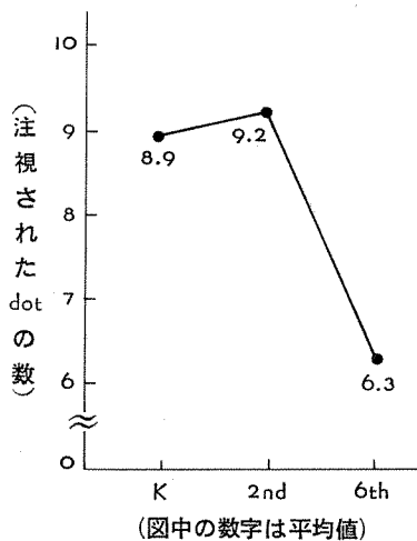
Fig. 7. 走査範囲
