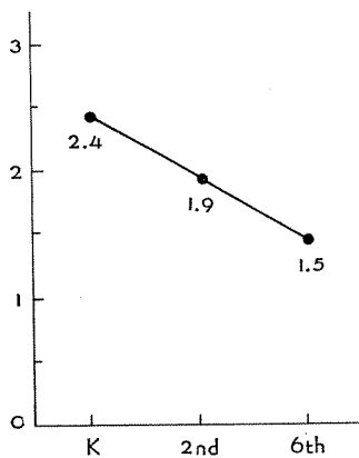
Fig. 8. 注視密度
