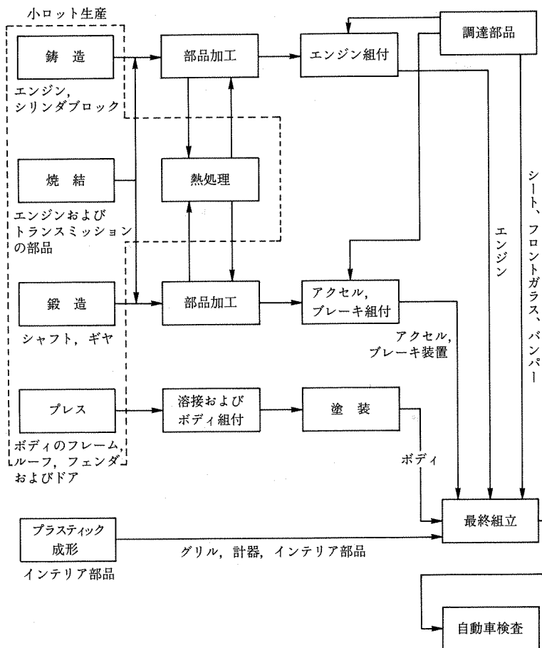
図2-1 T社の自動車製造工程
