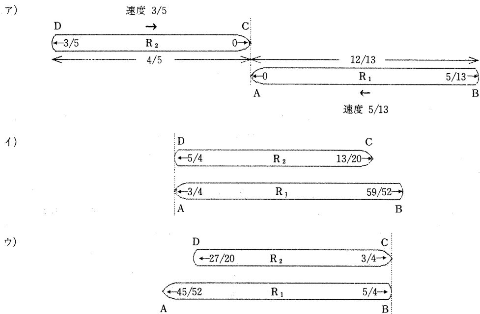
図3 2つのロケットのすれちがっていく様子③ (両方とも動いている場合)
