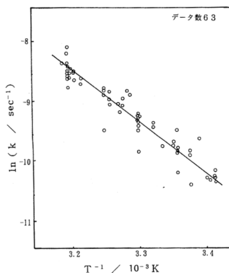
Fig. 2 改良した実験の結果
