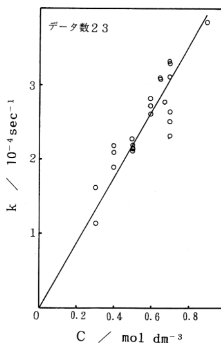
Fig. 4 酢酸メチルの塩酸触媒加水分解反応の 40 における速度定数 k と触媒濃度との関係
