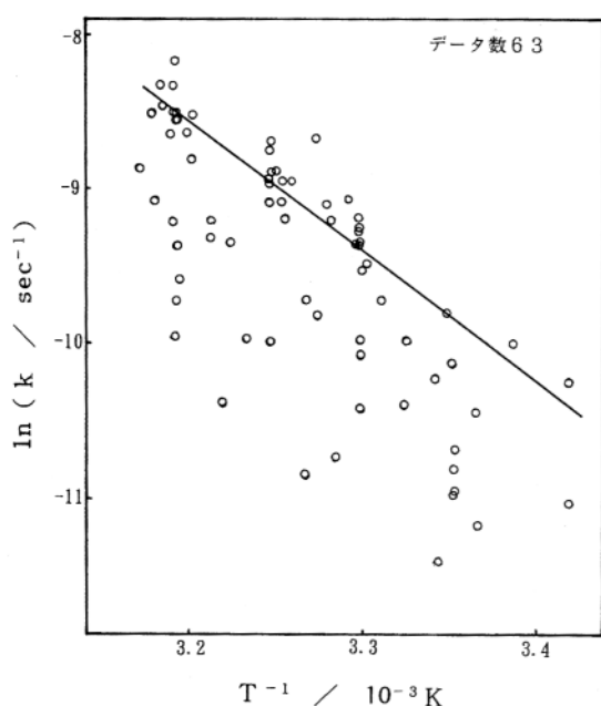
Fig. 1 テキスト (小笠原他 1986) に従った実験結果 (酢酸エチルの塩酸触媒加水分解反応のArrheniusプロット)
