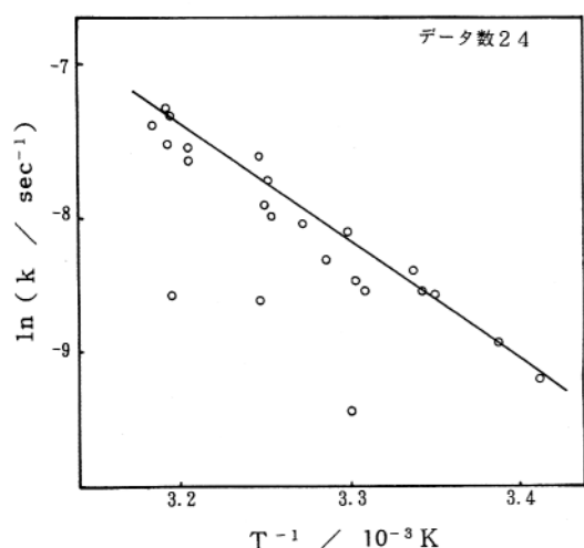
Fig. 3 改良した実験の結果 (ギ酸メチルの塩酸触媒加水分解反応のArrheniusプロット)
