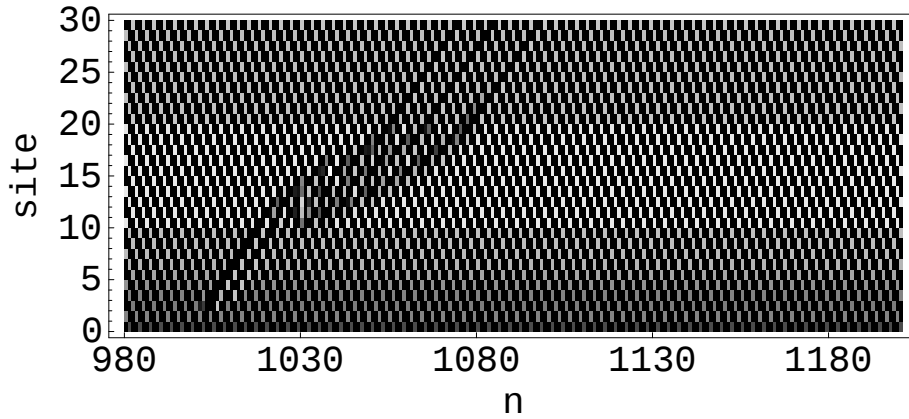
図2 各要素の状態変数 x_n^k \in [0.7, 2.3] を gray scale でプロットした時空間ダイアグラム．横軸が時間，縦軸が各要素の index を表す．3 番目の要素に入れたパルスが双方向領域 ( k = 11, \dots, 20 ) において加工されながら，下流領域 ( k = 21, \dots, 30 ) にまで伝達されている様子を表している．
