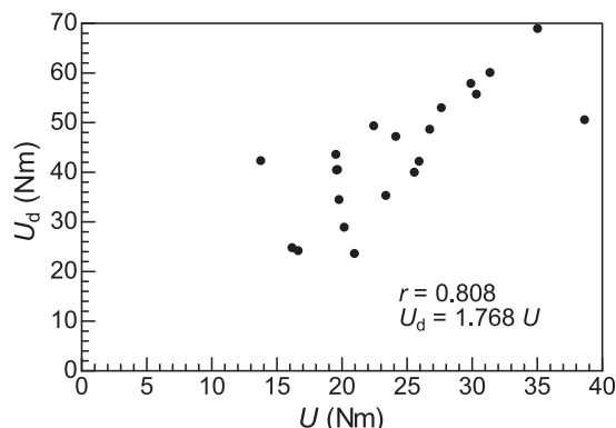
図5 静的曲げ破壊エネルギー ( U ) と衝撃曲げ吸収エネルギー ( U_d ) の関係 (各データは供試木平均値)
