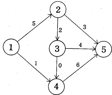
図9 例題(枝には運ぶべき荷物の量が表示されている。枝を通るトラック台数に制限はないとする)
