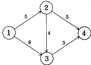
図3 最も簡単な例
