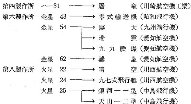
図3 三菱重工業発動機他社供給図
