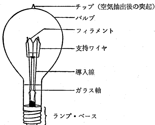
第 II-2-2 表 電球 各部 名称
