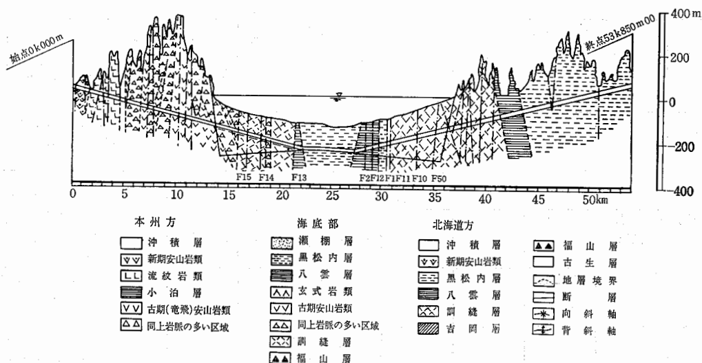
図 12 トンネルルート地質概要 縦断面図
