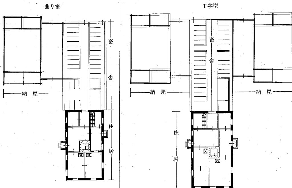
図 X-1 「曲り家」およびT字型農家見取図
