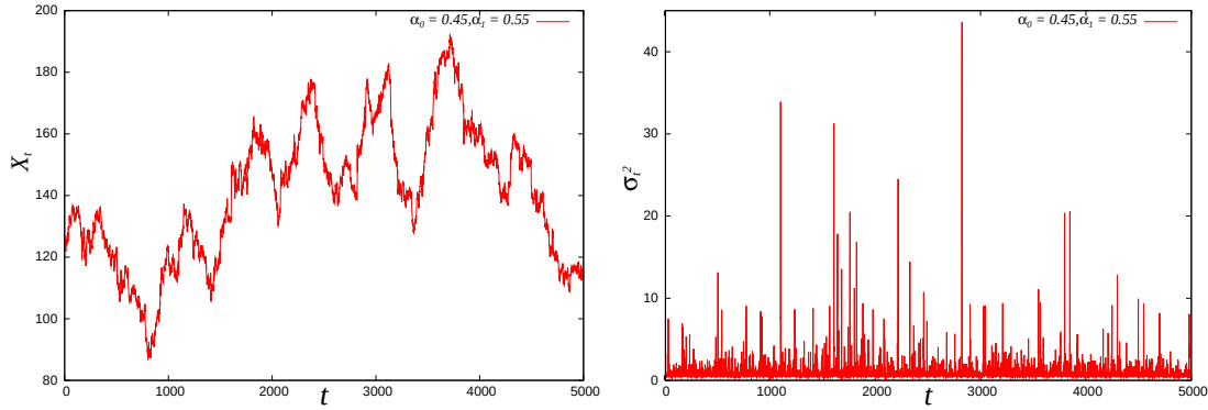
図 12: ARCH(1) 過程のレートの累積 X_t = \sum_{k=0}^{t-1} X_k (左) とボラティリティ \sigma_t^2 (右) の時間変化. ここではパラメータの値を \alpha_0 = 0.45, \alpha_1 = 0.55 と選んでいる.
