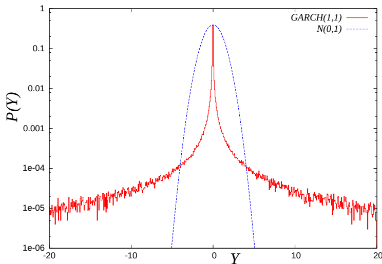
図 13: パラメータの値 (\alpha_0, \alpha_1, \beta_1) = (0.4, 0.3, 0.3) の場合 (尖度 \kappa = 4.17 ) の GARCH(1,1) 過程に対するリターン Y_t の分布. 比較のために \mathcal{N}(0, 1) も同時にプロットしてある.
