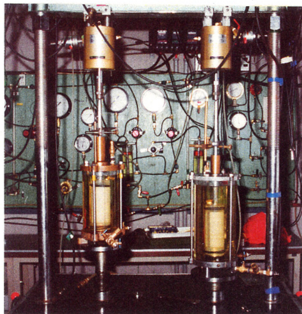
(d) conventional triaxial test apparatus
