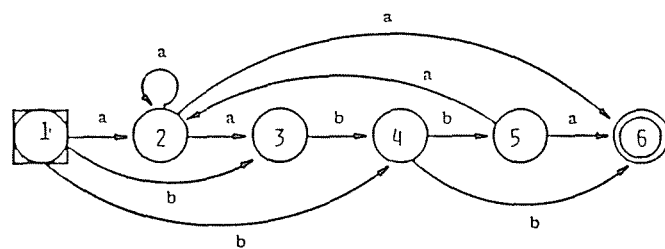
図 3. 5 (d) 例 3. 3 のオートマトン ( \wedge(1, 1) 法)
