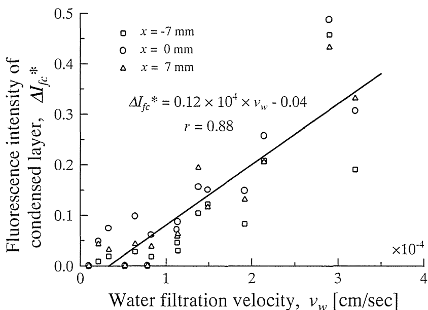
図 5-1 3. 濃縮蛍光強度におよぼす水透過速度の影響
