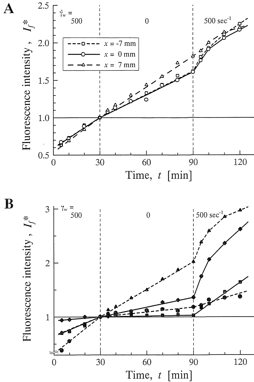
図 5 - 8. 蛍光強度におよぼす壁せん断速度の影響
