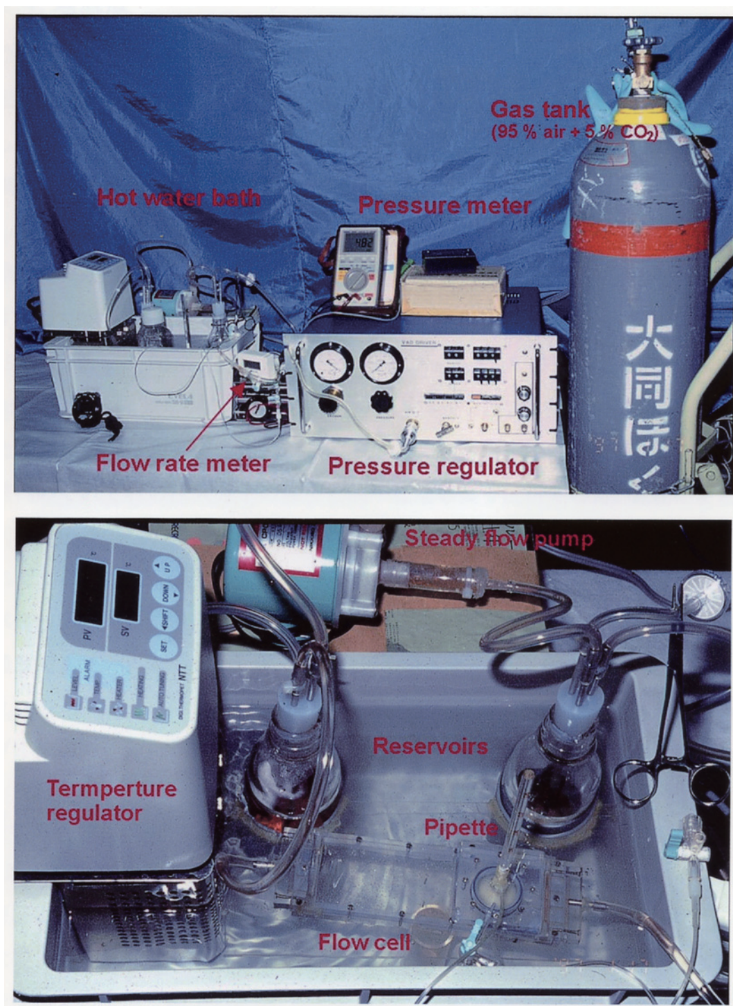
図3-3. 実験装置の外観写真
