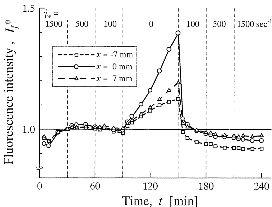
図 5-6. 血清を灌流液として用いた場合の蛍光強度におよぼす壁せん断速度の影響
