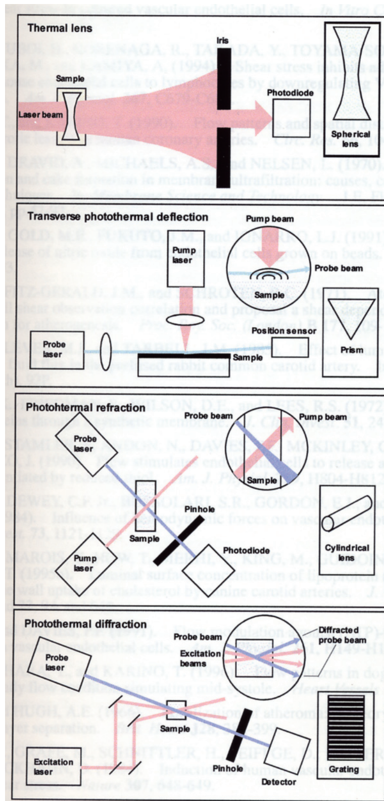
図2-6. 光熱レンズ法を用いる4つの測定原理 (from Morris and Peck, 1986)
