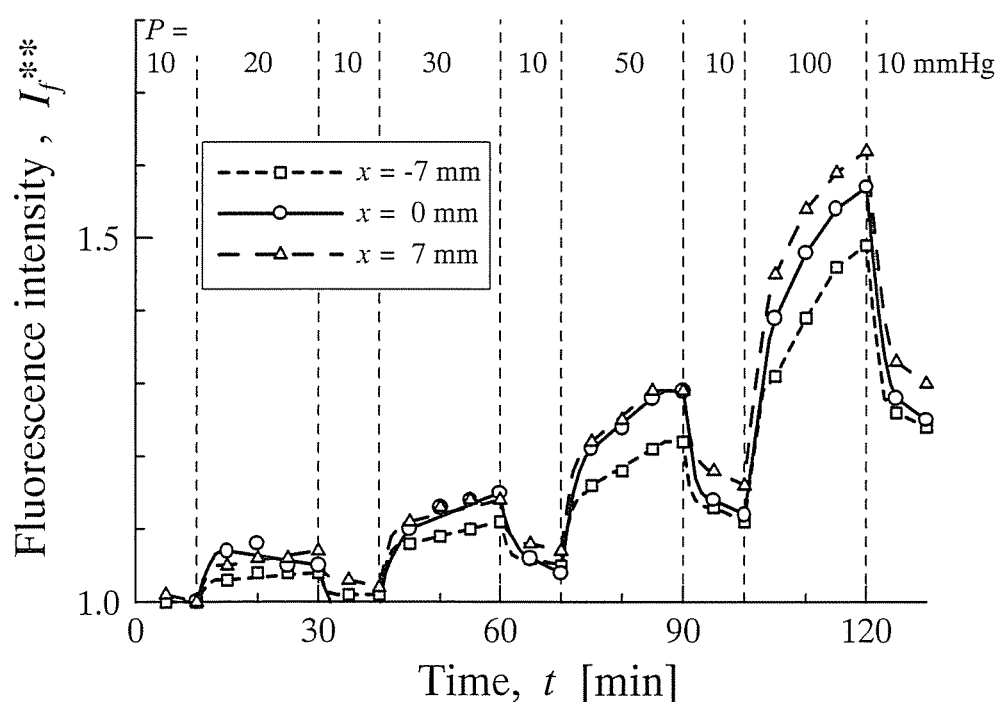
図5-2. 蛍光強度におよぼす圧力の影響
