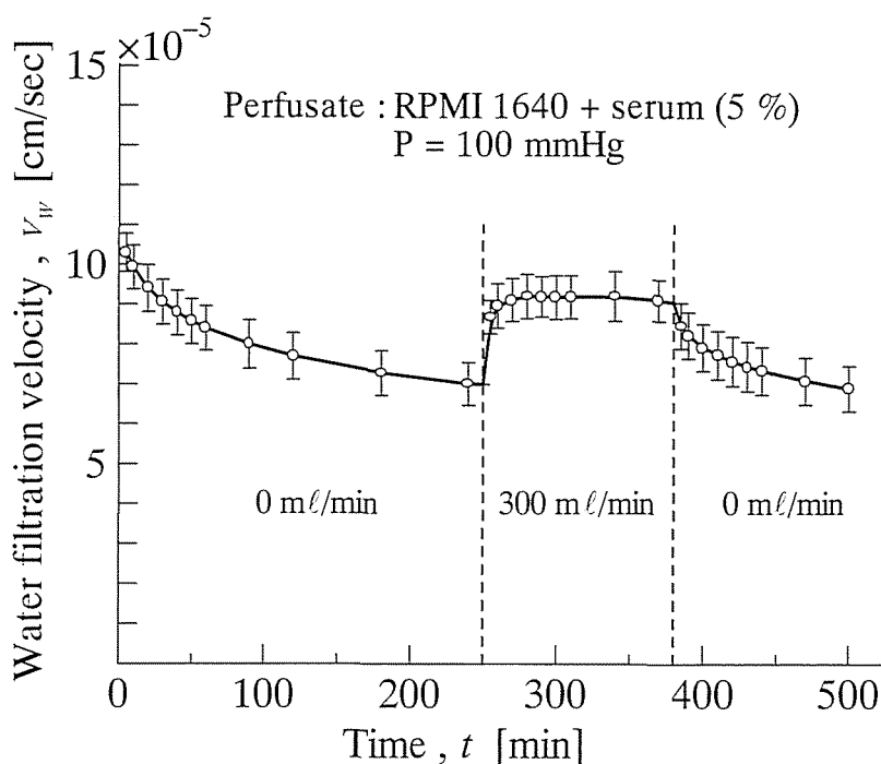
図4-6. 水透過速度におよぼす灌流流量の影響の可逆性
