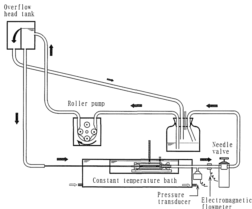
図4-2. 灌流装置の概略図
