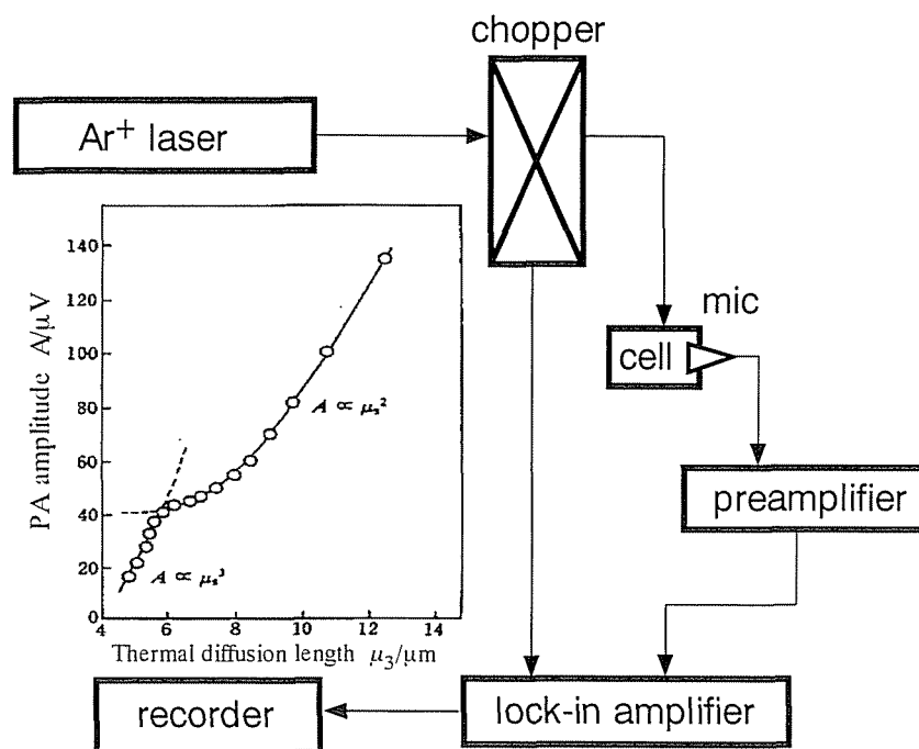
図2-5. 光音分光測定装置のブロックダイアグラム (from Hsueh et al., 1990)
