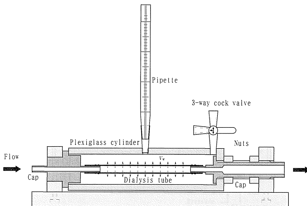
図4-1. 水透過速度測定装置の縦断面図
