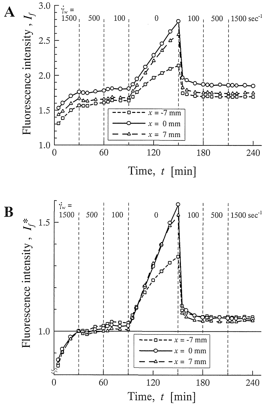
図 5-3. 蛍光強度におよぼす壁せん断速度の影響
