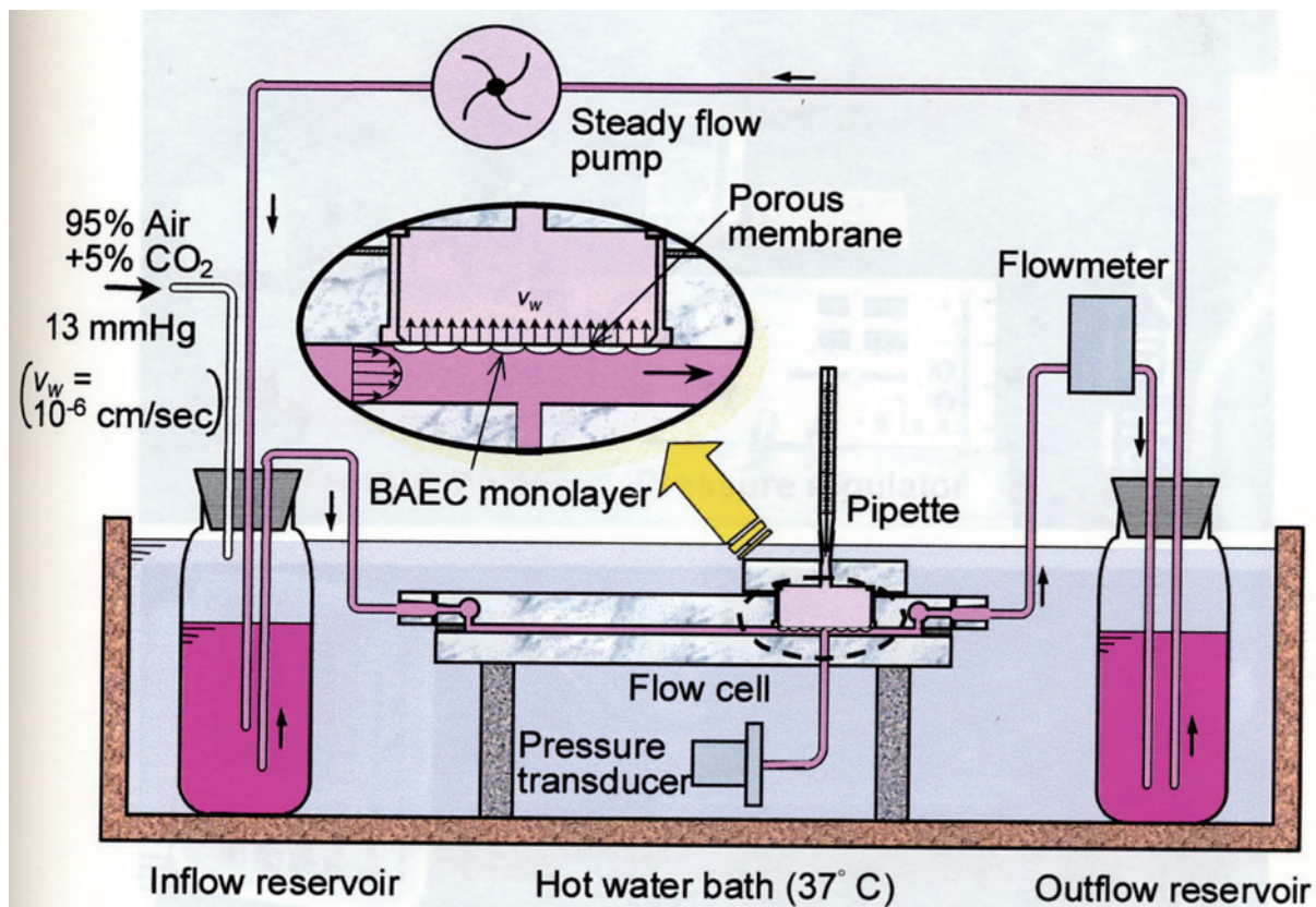
図3-2. 灌流装置の模式図
