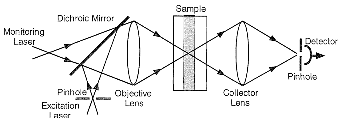
図 2-4. 顕微共焦点吸光分光法の光学系 (from Masuhara and Sasaki, 1995)
