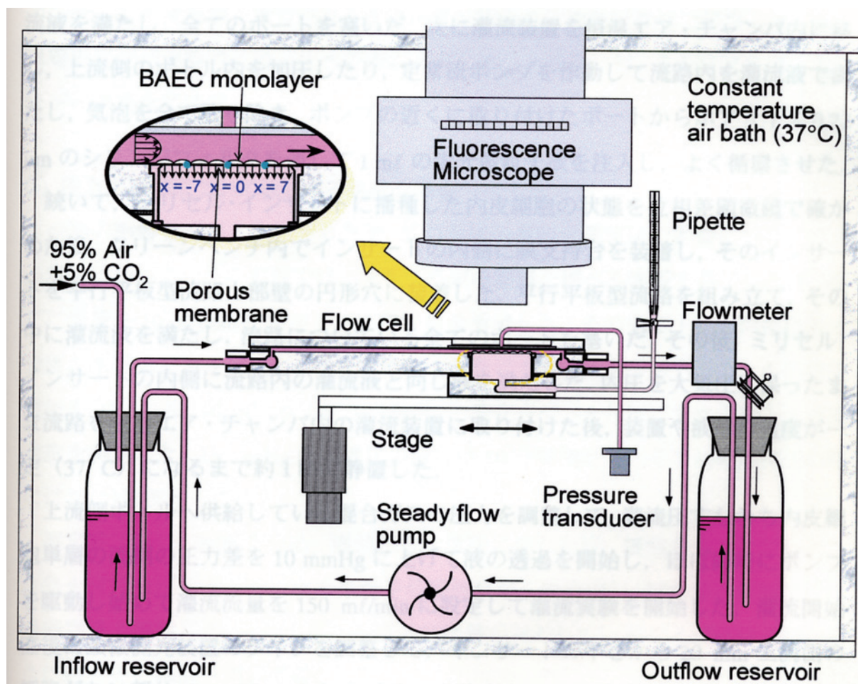
図 5-1. 灌流装置の模式図
