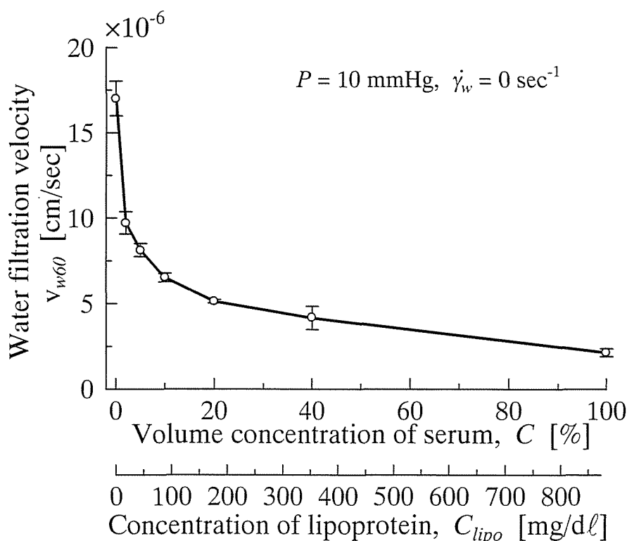
図3-4. 水透過速度におよぼす灌流液中の血清濃度の影響
