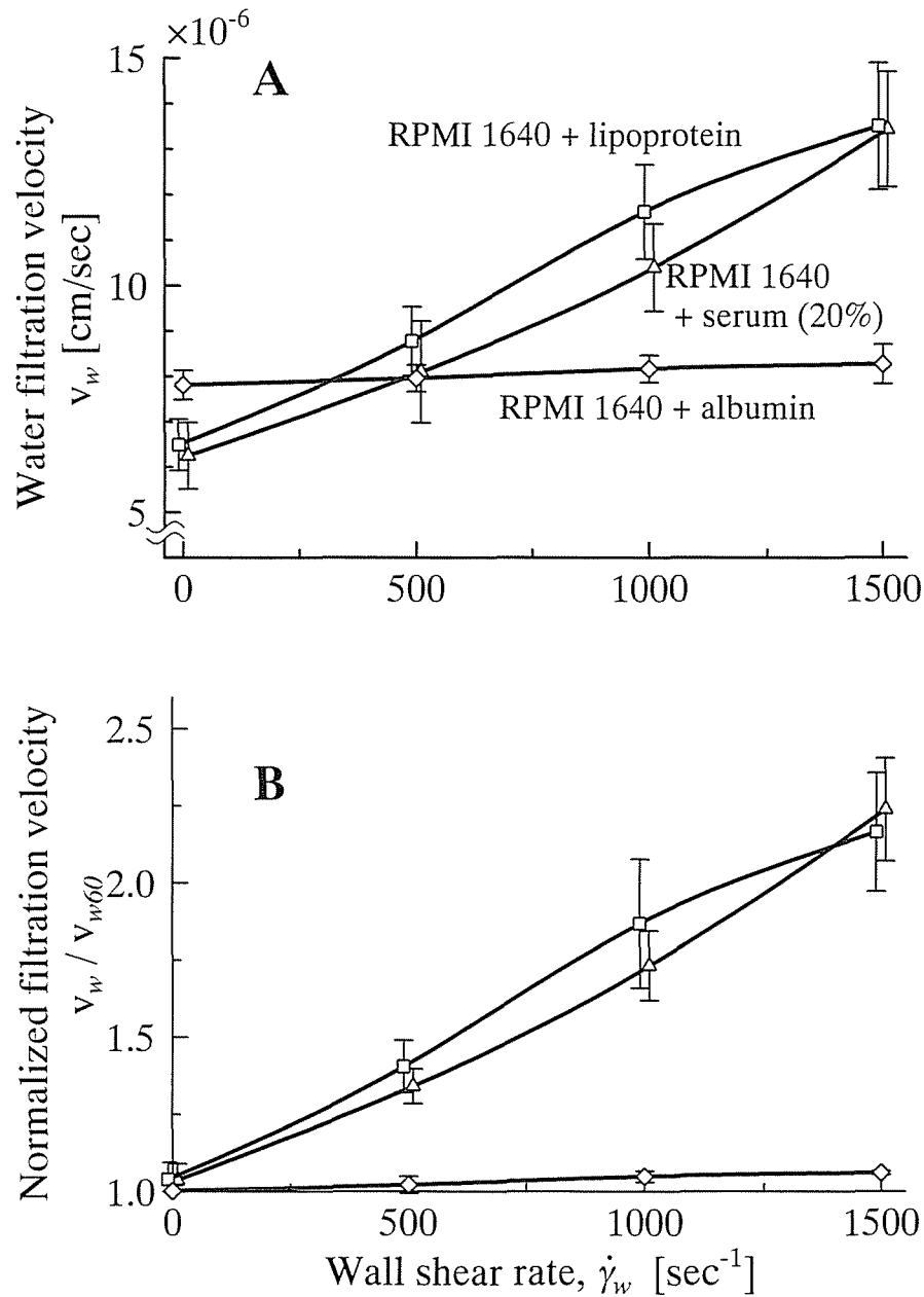
図3-9. リポ蛋白あるいはアルブミンのみを含んだ灌流液を用いた場合の水透過速度におよぼす壁せん断速度の影響
