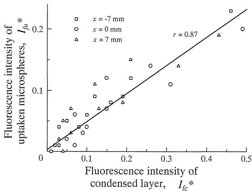
図 5-1 4. 濃縮蛍光強度と蓄積蛍光強度との関係
