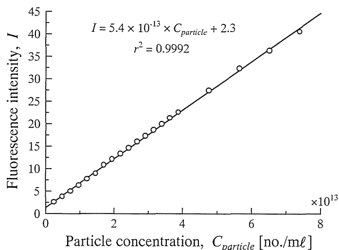
図 5 - 1 0 . 蛍光強度の較正線
