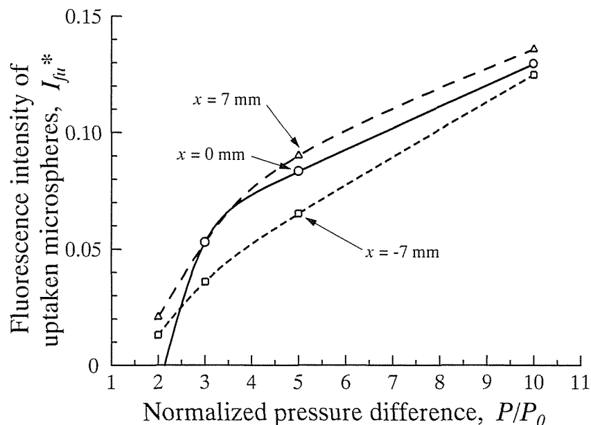
図 5-1 2. 蓄積蛍光強度におよぼす灌流圧の影響
