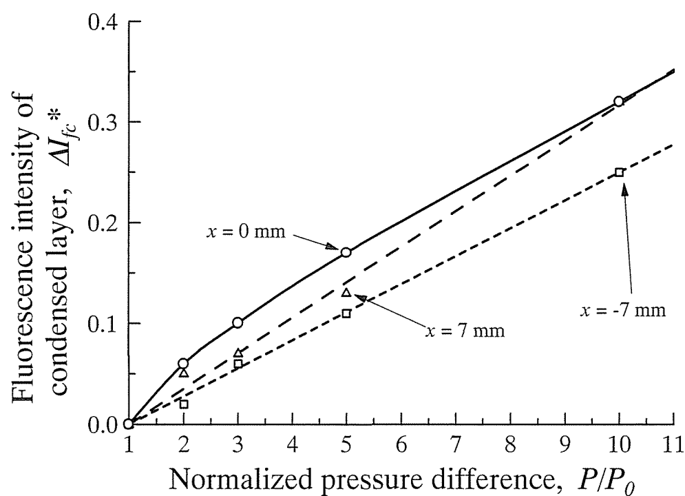
図 5 - 1 1 . 濃縮蛍光強度におよぼす灌流圧の影響
