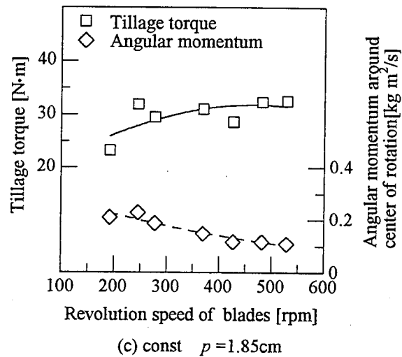
図6.3 平均耕うん軸トルグと耕うん軸まわりの角運動量
