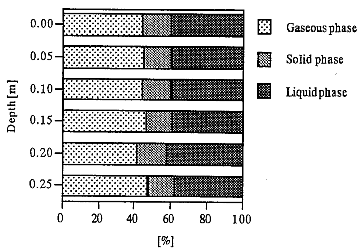
(b) アップカットロータリ耕
