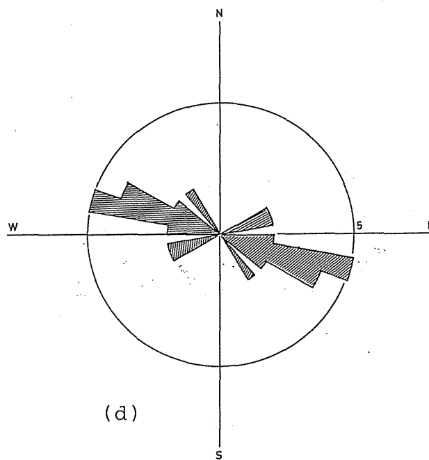
ARICA DIKE SWARM
