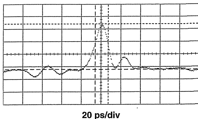
図 5.10 pin -PD のパルス応答
