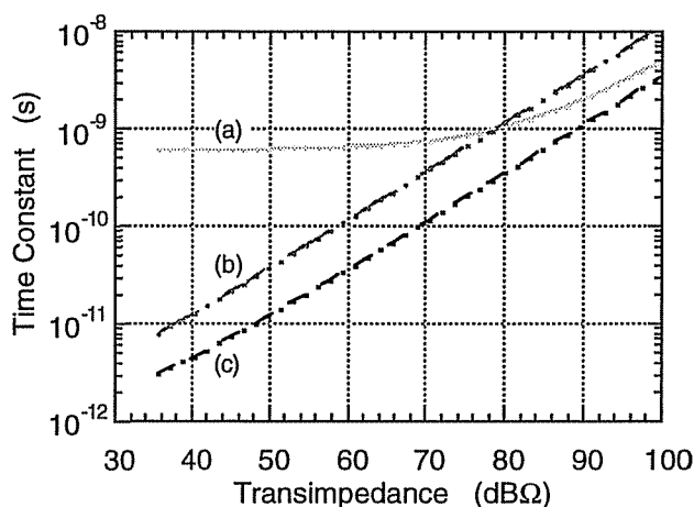
図 5.2 時定数とトランスインピーダンスの関係
