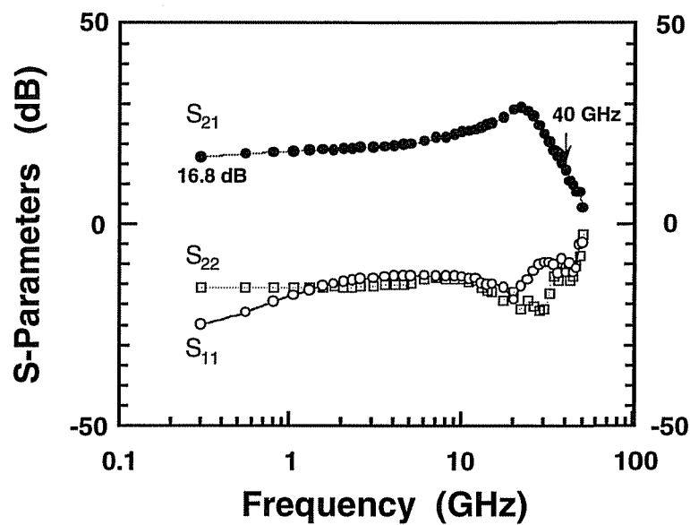
図 3.12 デバイス C の S パラメータの周波数特性
