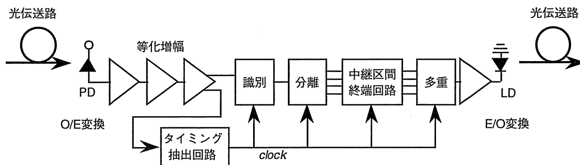
図1.3 中間中継器の構成例
