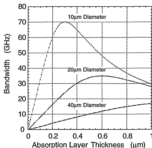
図 5.3 表面入射型 pin -PD の帯域と InGaAs 光吸収層の厚さの関係
