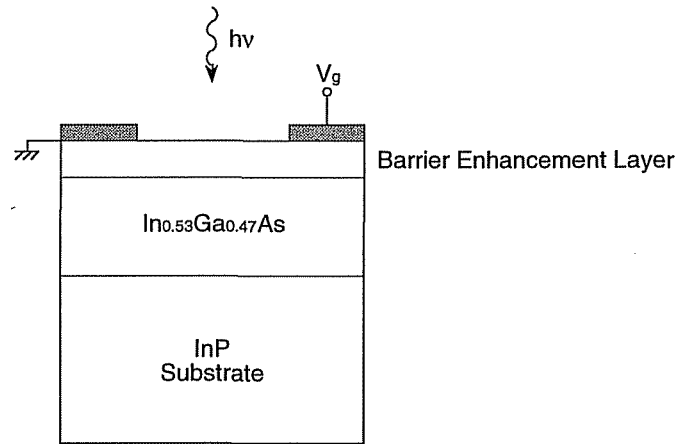
図 2.8 InGaAs MSM-PD のデバイス構造モデル
